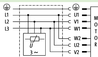
Varistor-suppression (triângulo)
